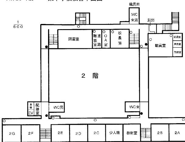
平成 28 年度 東中学校校舎平面図
