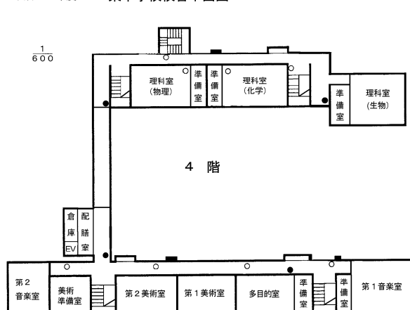
平成 27 年度 東中学校校舎平面図
